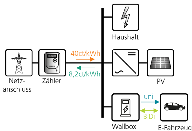
Abb. 2 schematische Darstellung des untersuchten Energiesystems Fraunhofer ISE
