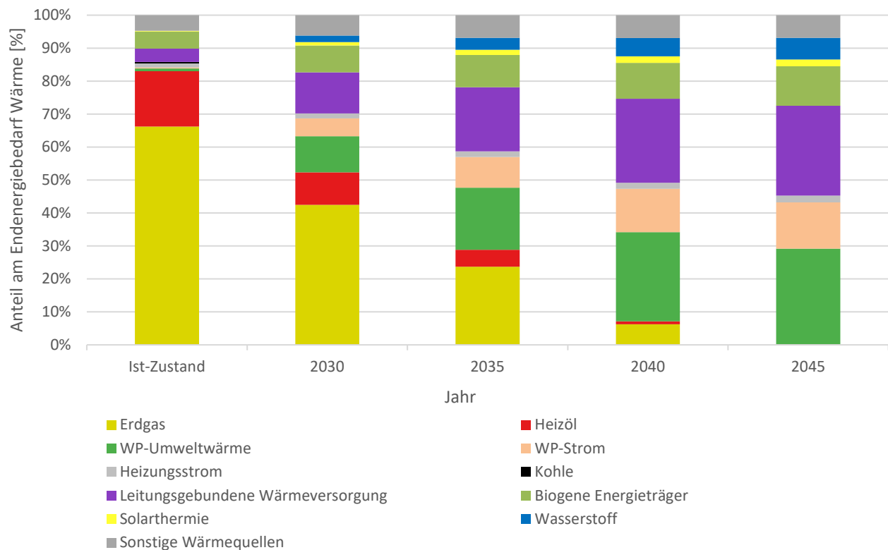
Abbildung 10: Entwicklung der Anteile der Energieträger am Endenergiebedarf Wärme der ausgewerteten KWP's - Kommunen mit mehr als 100.000 Einwohner*innen
