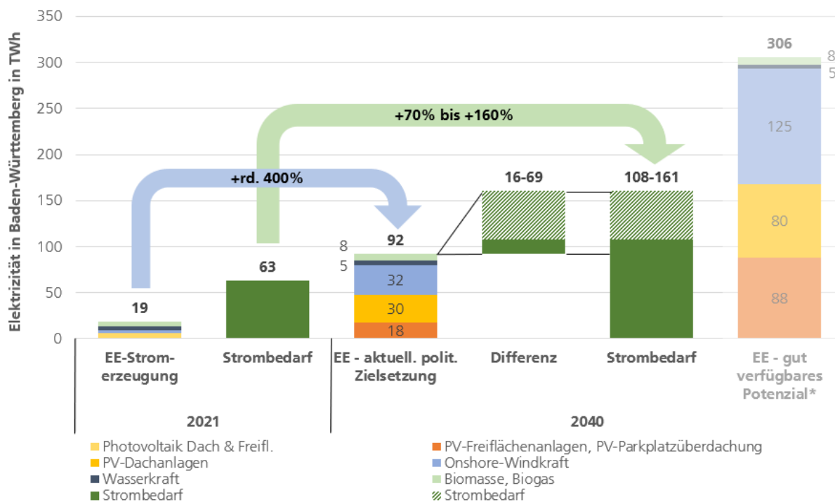
Abbildung 21: Heutige EE-Stromerzeugung und Strombedarf in Baden-Württemberg, Strombedarf und EE-Potenziale in 2040 7
