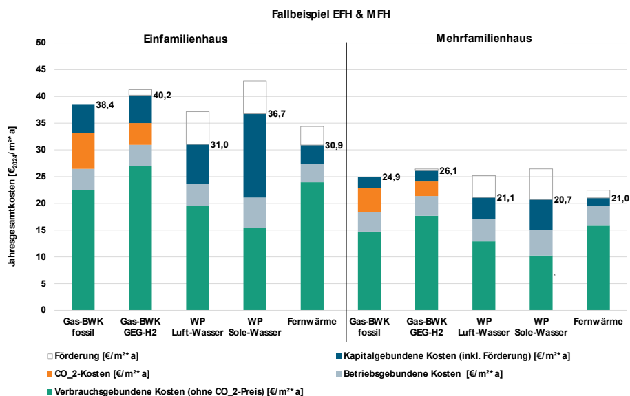
Abbildung 7: Sensitivität Heizkostenvergleich bei hohem CO 2 -Preisfad 20
