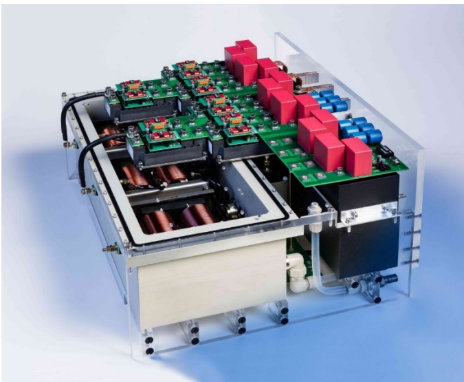
Hochkompakter Mittelspannungs-Wechselrichter mit SiC-Leistungsmodulen für Großspeicher und Verteilnetze, entwickelt im Projekt »SiC-MSBat«. © Fraunhofer ISE
