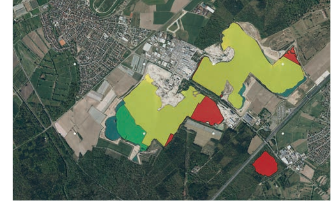
Beispiel für die Bestimmung des wirtschaftlich-praktischen Potenzials für schwimmende PV, spezifisch für jede Teilfläche des Sees berechnet.
