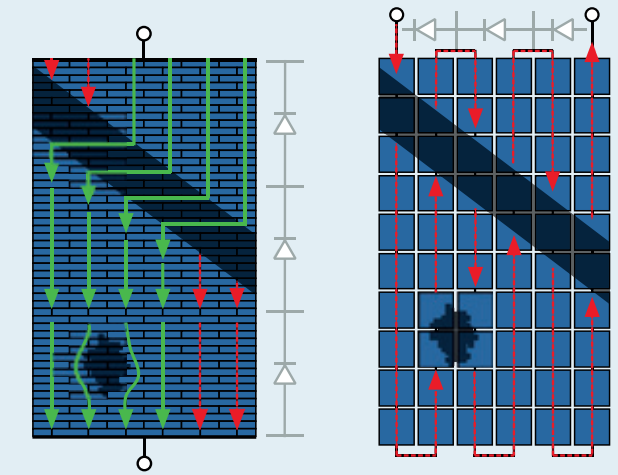
Links: Im Matrix-Schindelmodul kann der Strom verschattete Bereiche umfließen, rechts: im gewöhnlichen Modul wird der Stromfluss durch verschattete Bereiche unterbrochen.
