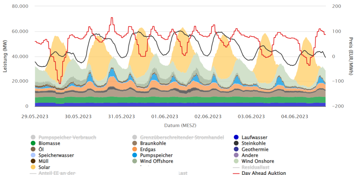
Abbildung 24: Beispiel für den Verlauf von Börsenstrompreisen, konventioneller und regenerativer Stromerzeugung der 22. Kalenderwoche 2023 [ISE4].
