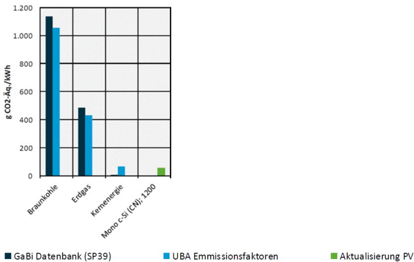
Abbildung 42: Treibhauspotenzial verschiedener Stromerzeugungstechnologien [UBA7].
