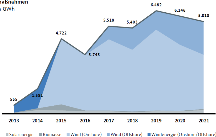
Abbildung 20: Abgeregelter elektrische Energie [BNA2].
