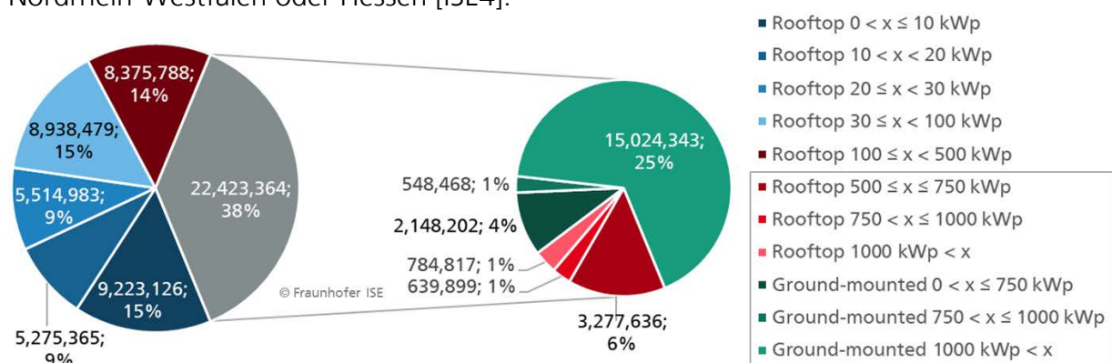
Abbildung 19: Verteilung der installierten PV-Leistung im Jahr 2021 nach Anlagengröße [ISE5].
