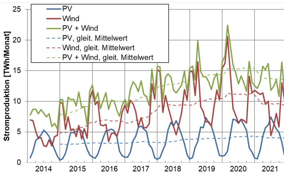
Abbildung 23: Monatssummen PV- und Windstromproduktion, Daten aus [ISE4].
