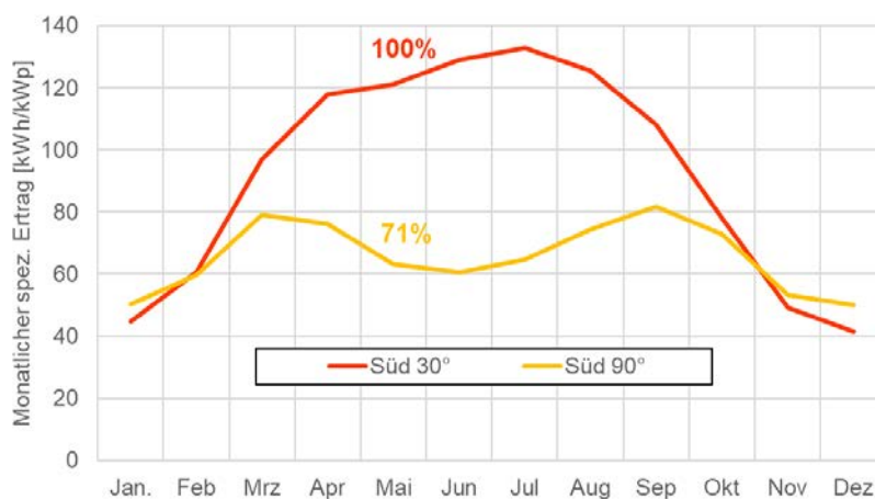
Abbildung 36: Monatliches, spezifisches Ertragspotenzial für verschiedene Neigungen, unverschattet, Standort Freiburg, berechnet online mit https://re.jrc.ec.europa.eu/pvg_tools/en/ ; die Prozentzahlen geben den relativen Jahresertrag bezogen auf 30° Neigung an.
