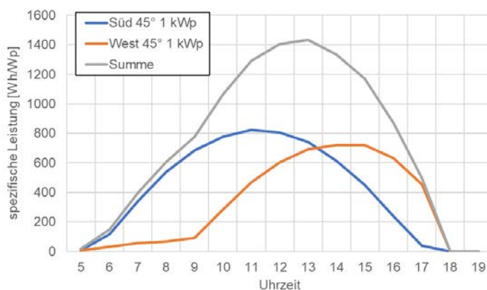
Abbildung 35: Stundenprofil der Stromproduktion an einem klaren Apriltag für verschiedene Dachausrichtungen bei 45° Dachneigung, unverschattet, Standort Freiburg, berechnet online mit https://re.jrc.ec.europa.eu/pvg_tools/en/ .
